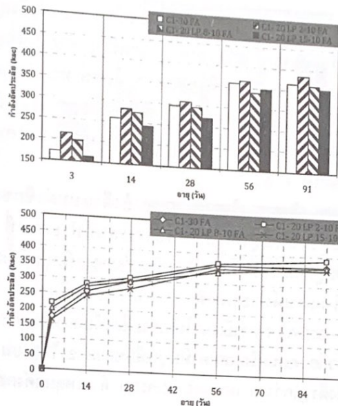
(ค) คอนกรีตผสมปูนซีเมนต์ปอร์ตแลนด์ประเภทที่ 1 ผงหินปูน และเถ้าลอย โดยทำการแทนที่ปอร์ตแลนด์ประเภทที่ 1 ด้วยผงหินปูนขนาด 2, 8 และ 15 ไมครอน ที่ร้อยละ 20 โดยน้ำหนักวัสดุผสม และเถ้าลอยร้อยละ 10 โดยน้ำหนักวัสดุผสม
