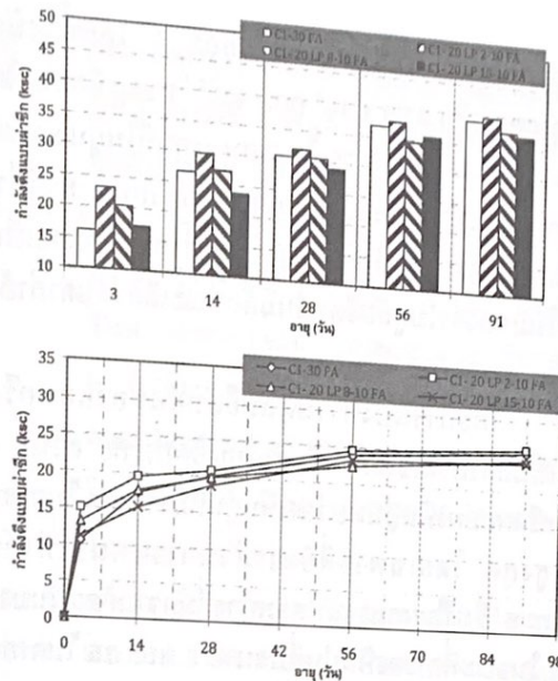
(ค) คอนกรีตผสมปูนซีเมนต์ปอร์ตแลนด์ประเภทที่ 1 ผงหินปูน และเถ้าลอย โดยทำการแทนที่ปอร์ตแลนด์ประเภทที่ 1 ด้วยผงหินปูนขนาด 2, 8 และ 15 ไมครอน ที่ร้อยละ 20 โดยน้ำหนักวัสดุผง และเถ้าลอยร้อยละ 10 โดยน้ำหนักวัสดุผง
