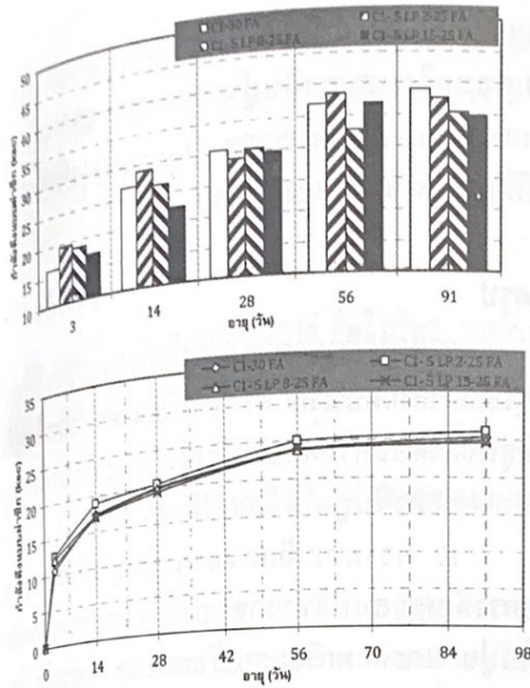
(ก) คอนกรีตผสมปูนซีเมนต์ปอร์ตแลนด์ประเภทที่ 1 ผงหินปูน และเถ้าลอย โดยทำการแทนที่ปอร์ตแลนด์ประเภทที่ 1 ด้วยผงหินปูนขนาด 2, 8 และ 15 ไมครอน ที่ร้อยละ 5 โดยน้ำหนักวัสดุผง และเถ้าลอยร้อยละ 25 โดยน้ำหนักวัสดุผง
