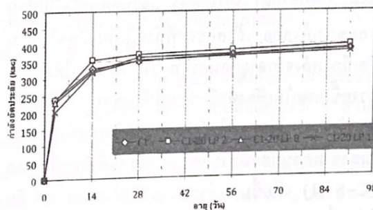
(ค) คอนกรีตผสมปูนซีเมนต์ปอร์ตแลนด์ประเภทที่ 1 และผงหินปูน โดยการแทนที่ปอร์ตแลนด์ประเภทที่ 1 ด้วยผงหินปูนขนาด 2, 8 และ 15 ไมครอน ที่ร้อยละ 20 โดยน้ำหนักวัสดุผสม
