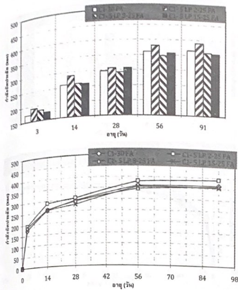
(ก) คอนกรีตผสมปูนซีเมนต์ปอร์ตแลนด์ประเภทที่ 1 ผงหินปูน และเถ้าลอย โดยทำการแทนที่ปอร์ตแลนด์ประเภทที่ 1 ด้วยผงหินปูนขนาด 2, 8 และ 15 ไมครอน ที่ร้อยละ 5 โดยน้ำหนักวัสดุผสม และเถ้าลอยร้อยละ 25 โดยน้ำหนักวัสดุผสม
