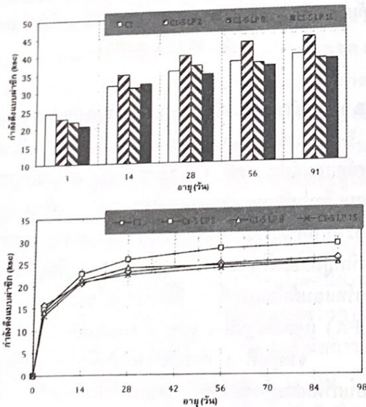
(ก) คอนกรีตผสมปูนซีเมนต์ปอร์ตแลนด์ประเภทที่ 1 และผงหินปูน โดยทำการแทนที่ปอร์ตแลนด์ประเภทที่ 1 ด้วยผงหินปูนขนาด 2, 8 และ 15 ไมครอน ที่ร้อยละ 5 โดยน้ำหนักวัสดุผง
