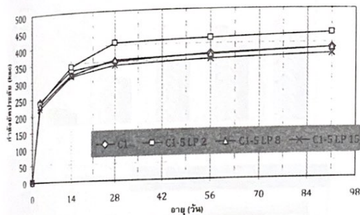
(ก) คอนกรีตผสมปูนซีเมนต์ปอร์ตแลนด์ประเภทที่ 1 และผงหินปูน โดยการแทนที่ปอร์ตแลนด์ประเภทที่ 1 ด้วยผงหินปูนขนาด 2, 8 และ 15 ไมครอน ที่ร้อยละ 20 โดยน้ำหนักวัสดุผสม
