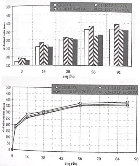
(ข) คอนกรีตผสมปูนซีเมนต์ปอร์ตแลนด์ประเภทที่ 1 ผงหินปูน และเถ้าลอย โดยทำการแทนที่ปอร์ตแลนด์ประเภทที่ 1 ด้วยผงหินปูนขนาด 2, 8 และ 15 ไมครอน ที่ร้อยละ 10 โดยน้ำหนักวัสดุผสม และเถ้าลอยร้อยละ 20 โดยน้ำหนักวัสดุผสม
