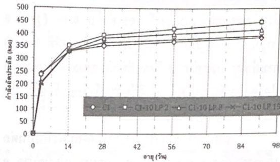
(ข) คอนกรีตผสมปูนซีเมนต์ปอร์ตแลนด์ประเภทที่ 1 และผงหินปูน โดยการแทนที่ปอร์ตแลนด์ประเภทที่ 1 ด้วยผงหินปูนขนาด 2, 8 และ 15 ไมครอน ที่ร้อยละ 10 โดยน้ำหนักวัสดุผสม
