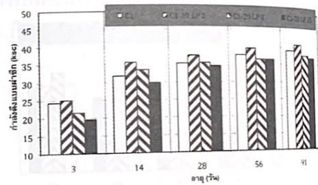
(ข) คอนกรีตผสมปูนซีเมนต์ปอร์ตแลนด์ประเภทที่ 1 และผงหินปูน โดยทำการแทนที่ปอร์ตแลนด์ประเภทที่ 1 ด้วยผงหินปูนขนาด 2, 8 และ 15 ไมครอน ที่ร้อยละ 10 โดยน้ำหนักวัสดุผง
