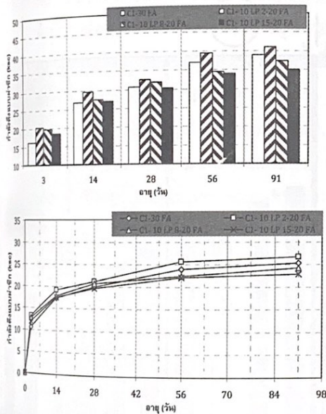
(ข) คอนกรีตผสมปูนซีเมนต์ปอร์ตแลนด์ประเภทที่ 1 ผงหินปูน และเถ้าลอย โดยทำการแทนที่ปอร์ตแลนด์ประเภทที่ 1 ด้วยผงหินปูนขนาด 2, 8 และ 15 ไมครอน ที่ร้อยละ 10 โดยน้ำหนักวัสดุผง และเถ้าลอยร้อยละ 20 โดยน้ำหนักวัสดุผง
