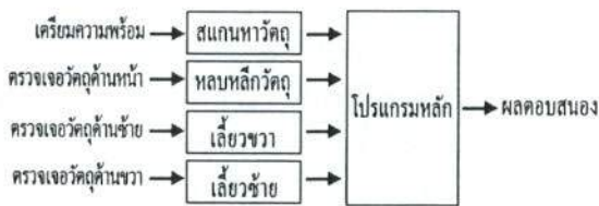
รูปที่ 2 แผนภาพแสดงพฤติกรรมของหุ่นยนต์ เพื่อทำการตัดสินใจ
