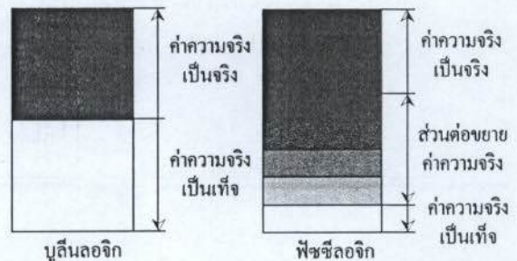
รูปที่ 1 ครรกะแบบจริงเท็จ (บูลีนลอจิก)
