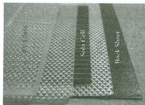
รูปที่ 1 วัสดุเคลือบประกอบแผงเซลล์แสงอาทิตย์
