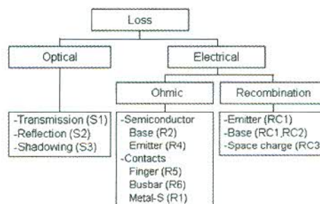
รูปที่ 9 พลังการสูญเสียกำลังไฟฟ้าของเซลล์แสงอาทิตย์
