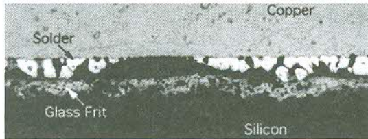
รูปที่ 10 เชื่อมต่อของเซลล์ (Silicon) กับลวดนำไฟฟ้า (Copper)
