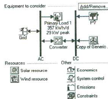
ภาพที่ 4.9 แบบจำลองระบบด้วยโปรแกรมคอมพิวเตอร์ HOMER
