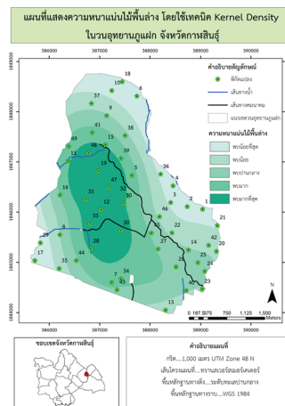
ภาพประกอบ 12 แสดงแผนที่ความหนาแน่น ไม้พื้นล่าง โดยใช้ Kernel Density
