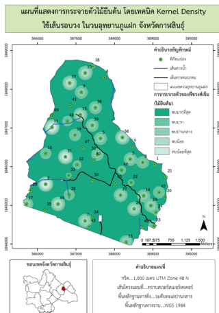
ภาพประกอบ 9 แสดงแผนที่การกระจายตัว ไม้ยืนต้น โดยใช้ Kernel Density
