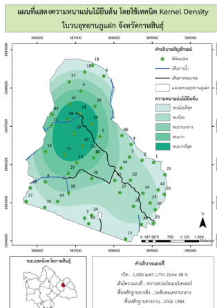
ภาพประกอบ 7 แสดงแผนที่ความหนาแน่นไม้ยืนต้น โดยใช้ Kernel Density
