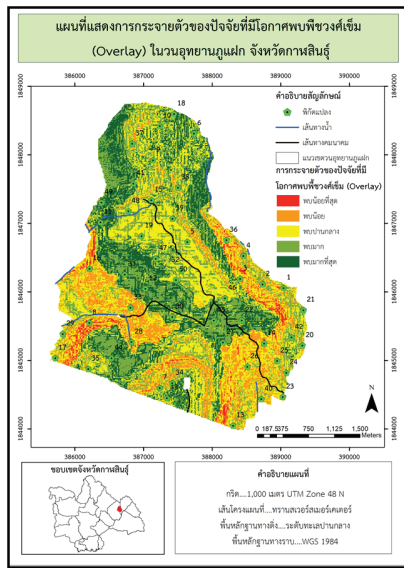
ภาพประกอบ 14 แผนที่แสดงผลการวิเคราะห์ปัจจัยด้วยการซ้อนทับที่มีโอกาสพบพืชวงศ์เข็ม
