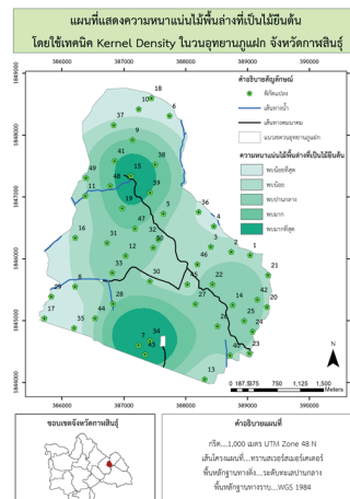
ภาพประกอบ 10 แสดงแผนที่ความหนาแน่นไม้ พื้นล่างที่เป็นไม้ยืนต้น โดยใช้ Kernel Density
