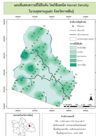
ภาพประกอบ 8 แสดงแผนที่ความถี่ไม้ยืนต้น โดยใช้ Kernel Density
