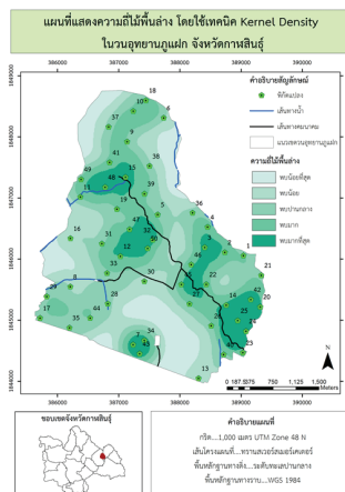
ภาพประกอบ 13 แสดงแผนที่ความถี่ไม้พื้นล่าง โดยใช้ Kernel Density
