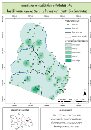
ภาพประกอบ 11 แสดงแผนที่ความถี่ไม้พื้นล่าง ที่เป็นไม้ยืนต้น โดยใช้ Kernel Density
