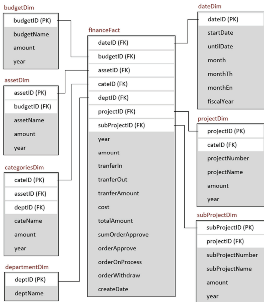
ภาพประกอบ 4 Star schema ของฐานข้อมูล OLAP
