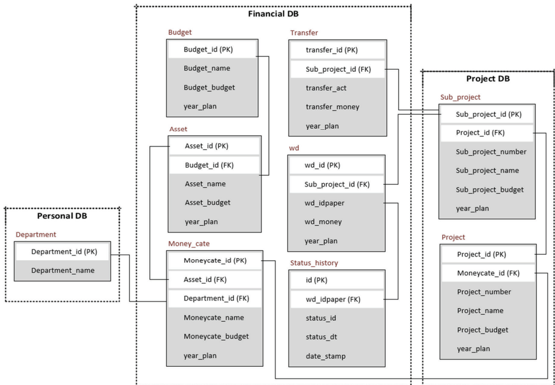
ภาพประกอบ 3 ER-Diagram ของฐานข้อมูล OLTP
