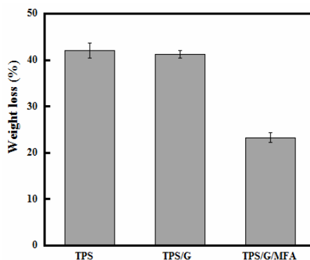
ภาพที่ 3 น้ำหนักที่หายไปของพลาสติกชีวภาพจากแป้ง พลาสติกชีวภาพจากแป้งผสมกลูเตนข้าวสาลี พลาสติกชีวภาพจากแป้งผสมกลูเตนข้าวสาลี และเข้ากับยางบด ที่ทำการทดสอบการเสื่อมสภาพด้วยเครื่องเร่งสภาวะเป็นเวลา 192 ชั่วโมง
