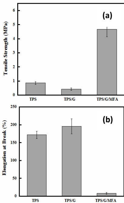
ภาพที่ 1 ค่าความต้านทานแรงดึง (a) และระยะยืด ณ จุดขาด (b) ของพลาสติกชีวภาพจากแป้ง (TPS) พลาสติกชีวภาพจากแป้งผสมกลูเตนข้าวสาลี (TPS/G) และพลาสติกชีวภาพจากแป้งผสมกลูเตนข้าวสาลีและแป้งไม่ยวบ (TPS/G/MFA)
