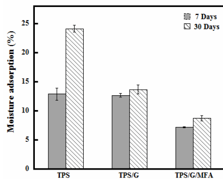
ภาพที่ 2 ค่าการดูดซับความชื้นของพลาสติกชีวภาพจากแป้ง พลาสติกชีวภาพจากแป้งผสมกลูเตนข้าวสาลีและพลาสติกชีวภาพจากแป้งผสมกลูเตนข้าวสาลีและแป้งไม่ยวบ ที่ทำการทดสอบภายหลังจากเก็บตัวอย่างเป็นเวลา 7 และ 30 วัน
