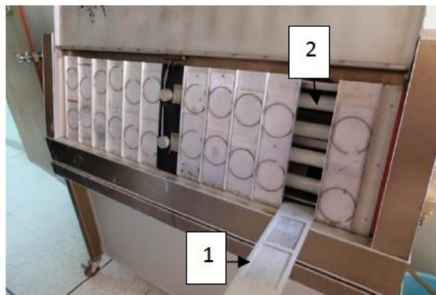
ภาพที่ 1 เครื่องเร่งสภาวะQUV รุ่นQUV/SE ขณะเปิดฝาครอบ
