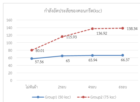
ภาพที่ 8 กำลังอัดประลัยของคอนกรีตเมื่อเสริมกำลังโดยวิธีการพันผ้าในแต่ละรอบ
