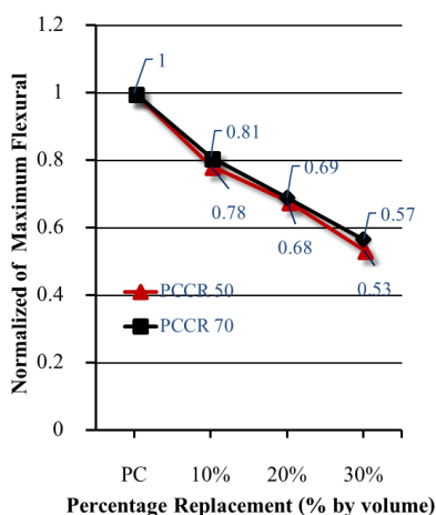
ภาพที่ 5 แสดงอัตราส่วนกำลังดัด คอนกรีตผสมเม็ดยางเคลือบพลาสติก PCCR 50 และ PCCR 70
