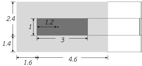
รูปที่ 1 ขนาดสายอากาศไมโครสตริป
