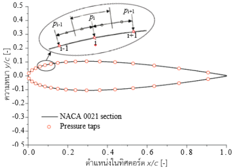
รูปที่ 7 แผนอากาศ NACA0021 และตำแหน่งวัดความดัน
