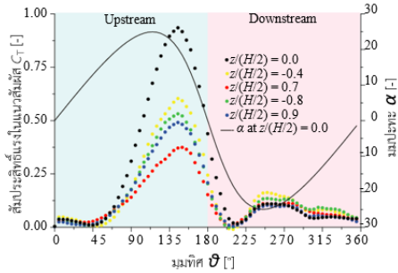
รูปที่ 11 ความผันผวนของสัมประสิทธิ์แรงในแนวสัมผัสกับมุมทิศ (ตำแหน่ง z/(H/2) = -0.8, -0.4, 0.0, 0.7 และ 0.9, ที่ \lambda=2.37 )
