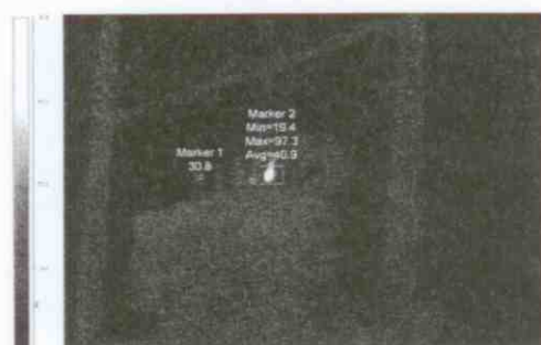
รูปที่ 4 จุดต่อบริเวณบัสซึ่งด้านทุติยภูมิของหม้อแปลงไฟฟ้าพิกัด 500 kVA เข้า โรงงานอุตสาหกรรม
