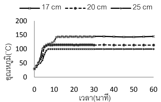
รูปที่ 5 การเปลี่ยนแปลงอุณหภูมิไอน้ำ
