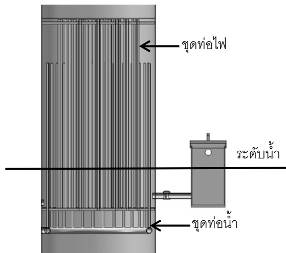
รูปที่ 4 ชุดท่อน้ำ ชุดท่อไฟและ การวัดระดับการเติมน้ำ
