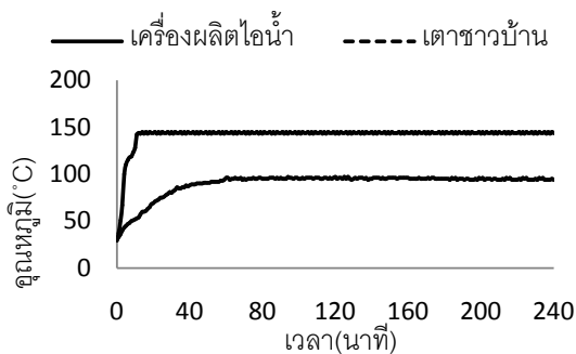
รูปที่ 6 การเปลี่ยนแปลงอุณหภูมิไอน้ำของเครื่องผลิตไอน้ำความดันต่ำและเตาแบบชาวบ้าน
