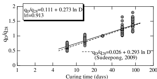
รูปที่ 6 ความสัมพันธ์ระหว่างกำลังอัดแกนเดียวและอายุบ่มภายใต้สภาวะตัวแปรต่างๆและการ Normalization
