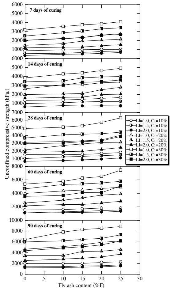
รูปที่ 3 ความสัมพันธ์ระหว่างกำลังอัดและปริมาณเถ้าลอยของดินซีเมนต์เถ้าลอยที่อายุบ่มต่างๆ
