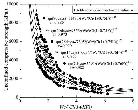
รูปที่ 4 ความสัมพันธ์ระหว่างกำลังอัดและปริมาณน้ำในดินต่อปริมาณปูนซีเมนต์
