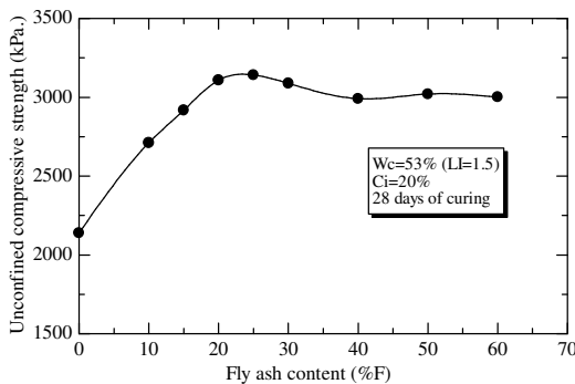
รูปที่ 2 กำลังอัดแกนเดียวของดินซีเมนต์เถ้าลอยผ่านหินที่อายุบ่ม 28 วัน
