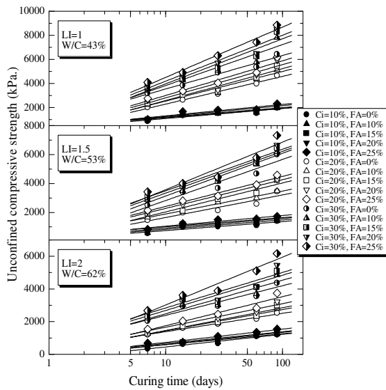
รูปที่ 5 ความสัมพันธ์ระหว่างกำลังอัดแกนเดียวและอายุบ่ม ของดินซีเมนต์เถ้าลอย
