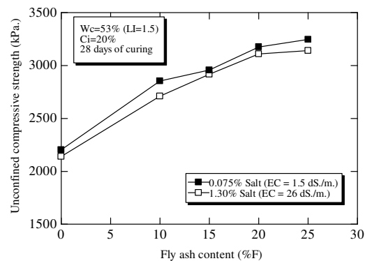
รูปที่ 1 อิทธิพลของความเค็มต่อกำลังอัดแกนเดียวของดินเค็มซีเมนต์เถ้าลอยถ่านหิน ที่อายุบ่ม 28 วัน
