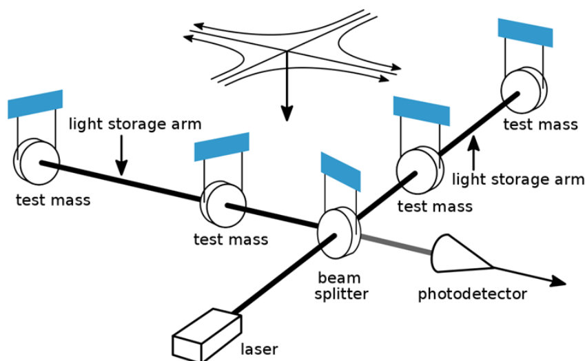
รูปที่ 5 แผนภาพอย่างง่ายที่แสดงให้เห็นถึงการทำงานของ interferometer ของ LIGO โดยคลื่นความโน้มถ่วงเมื่อเคลื่อนที่มาจากด้านบน ดังภาพ จะทำให้ความยาวแขนของเครื่องวัดเปลี่ยนแปลงไป ความเปลี่ยนแปลงสามารถอ่านได้จากริ้วของการแทรกสอดที่เกิดขึ้น (เครดิตภาพ Wikimedia Commons)
