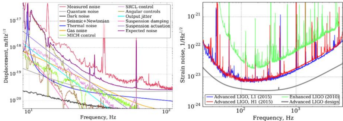
รูปที่ 6 ภาพด้านซ้าย เป็นสัญญาณรบกวนที่เกิดจากฟิสิกส์ที่แตกต่างกัน ดังที่แสดงเป็นเส้นสีต่าง ๆ เมื่อรวมสัญญาณรบกวนทุกอันเข้าด้วยกันจะได้เส้น expected noise ที่จะบอกถึงความไวของเครื่องวัด LIGO , ภาพด้านขวา แสดงความไวของเครื่อง LIGO กล่าวคือ เครื่องจะวัดได้ก็ต่อเมื่อสัญญาณ strain มีค่ามากกว่าเส้นผลรวมของสัญญาณรบกวน จากภาพจะเห็นว่าเครื่องจะวัดได้ไวที่สุดช่วง 100-1,000 Hz ซึ่ง aLIGO ถูกออกแบบให้วัด strain ได้เล็กกว่า 10^{-23} เลยทีเดียว (เครดิตภาพ [12] )
