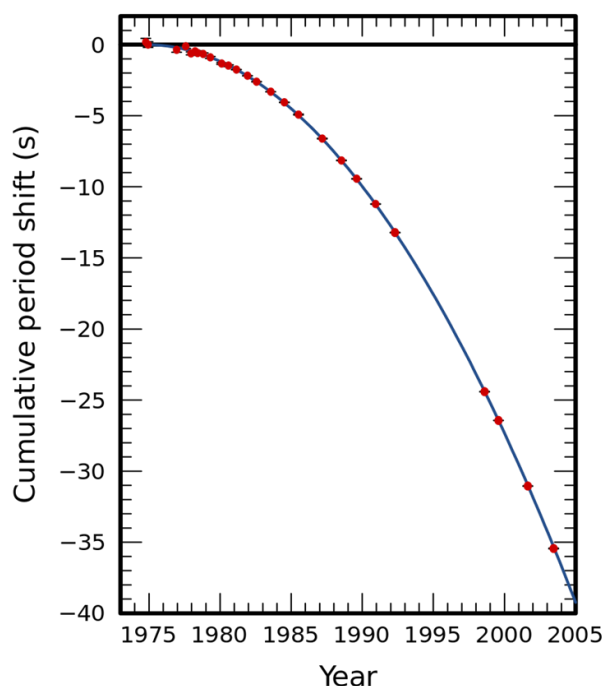
รูปที่ 3 แสดงการสูญเสียพลังงานของวงโคจรระบบพัลซาร์คู่ PSR 1913+16 โดยพล็อต การเลื่อนไปสะสม ของ epoch of periastron ที่สังเกตได้ในปีต่าง ๆ เทียบกับทฤษฎีสัมพัทธภาพทั่วไป บางช่วงที่จุดห่างเกิดจากการบีบอัดเกรคของกล้องโทรทรรศน์ การเก็บข้อมูลเป็นระยะเวลา 30 ปี พบว่าผลการสังเกตการณ์สอดคล้องกับทฤษฎีคลื่นความโน้มถ่วงเป็นอย่างดี (เครดิตภาพ [8])
