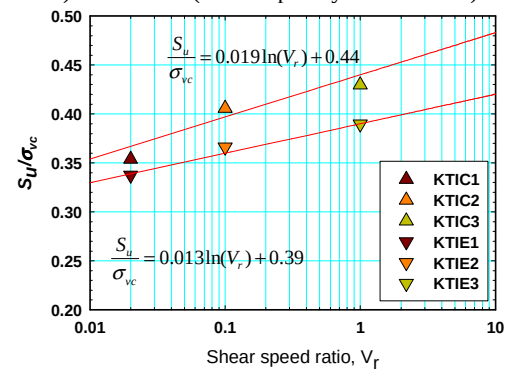
c) DSB test
