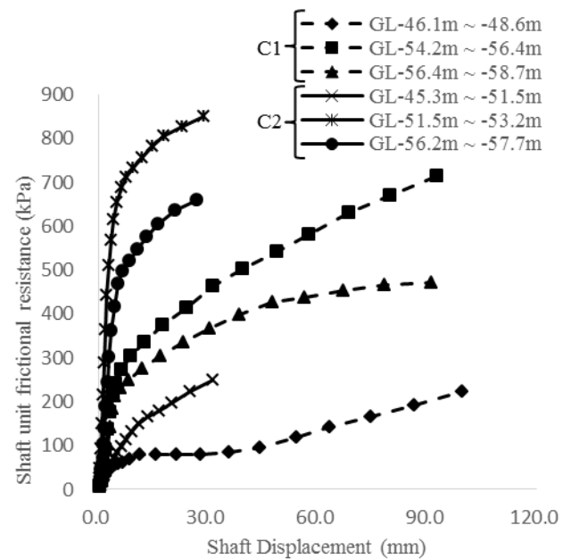
(b) IGM layer
