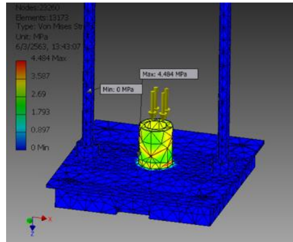
รูปที่ 5 ความเค้นจากการรับแรงที่กระทำกับแม่พิมพ์ตัวบน
