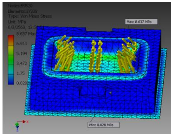
รูปที่ 6 ความเค้นจากการรับแรงที่กระทำกับแม่พิมพ์ตัวเมีย
