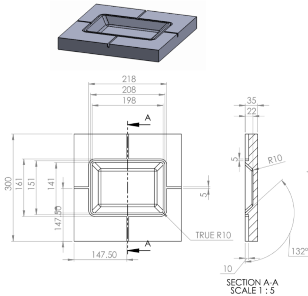
รูปที่ 3 แบบแม่พิมพ์ตัวล่าง
