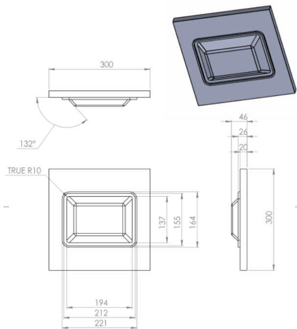
รูปที่ 4 แบบแม่พิมพ์ตัวบน
