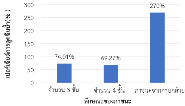
รูปที่ 13 กราฟการเปรียบเทียบเปอร์เซ็นต์การดูดซึมน้ำ
