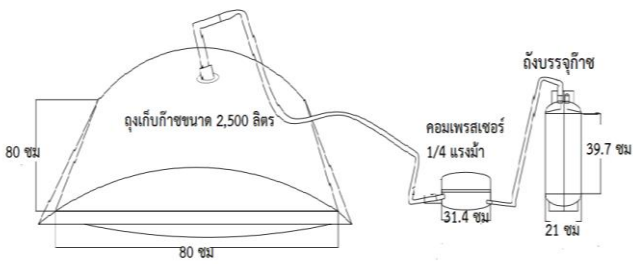
รูปที่ 1 แบบจำลองชุดทดลองในการอัดและเก็บก๊าซชีวภาพ
