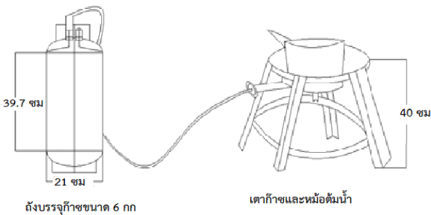
รูปที่ 2 แบบจำลองชุดทดลองการหาค่าความร้อน
