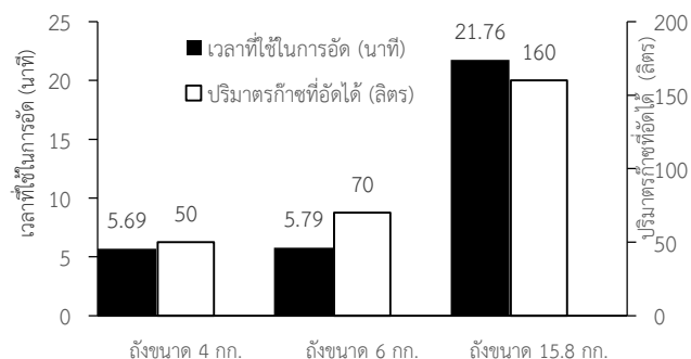
รูปที่ 5 เวลาที่ใช้ในการอัดและปริมาตรก๊าซชีวภาพที่อัดได้
