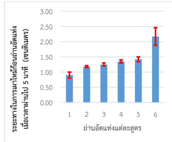
รูปที่ 8 ระยะทางในการเผาไหม้ของถ่านอัดแท่งสูตรต่าง ๆ เมื่อเวลาผ่านไป 5 นาที
