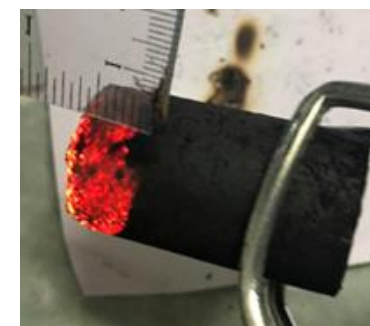
รูปที่ 11 ระยะทางการเผาไหม้ของก้อนถ่านอัดแท่งแบบผสมแอลกอฮอล์แข็ง สูตรที่ 3 เมื่อเวลาผ่านไป 5 นาที
