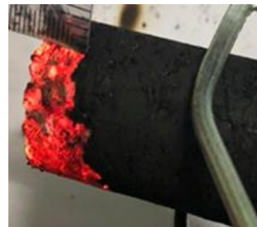
รูปที่ 10 ระยะทางการเผาไหม้ของก้อนถ่านอัดแท่งแบบผสมแอลกอฮอล์แข็ง สูตรที่ 2 เมื่อเวลาผ่านไป 5 นาที
