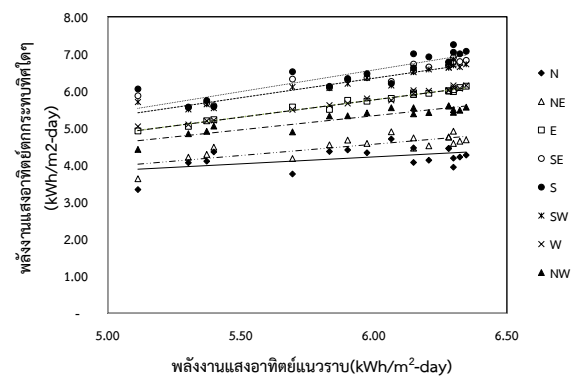
รูปที่ 4 ความสัมพันธ์ระหว่างพลังงานแสงอาทิตย์แนวราบ ( E_T ) กับพลังงานแสงอาทิตย์ที่ทิศต่างๆที่มุม 40 องศา( E_{xx40} )
