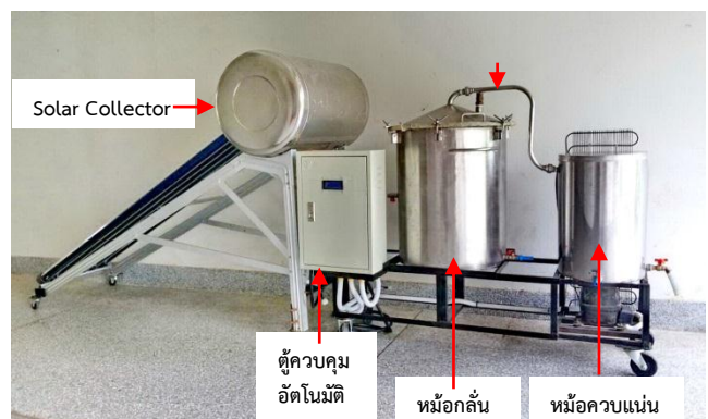
รูปที่ 13 การสร้างเครื่องกลั่นน้ำมันหอมระเหยสมุนไพรร่วมกับตัวเก็บรังสีแสงอาทิตย์
