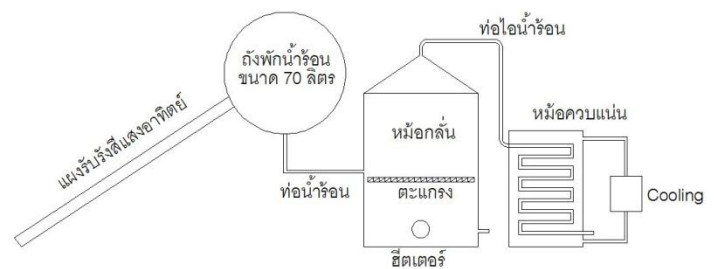
รูปที่ 9 ส่วนประกอบของเครื่องกลั่นน้ำมันหอมระเหย
