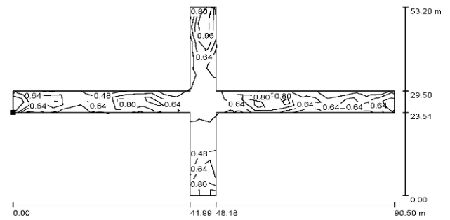
รูปที่ 25 ระดับความส่องสว่าง (Isolines of luminance, L_{av} ) หน่วยเป็น ( \text{cd}/\text{m}^2 ) บริเวณที่ 4 ทาง 4 แยก
