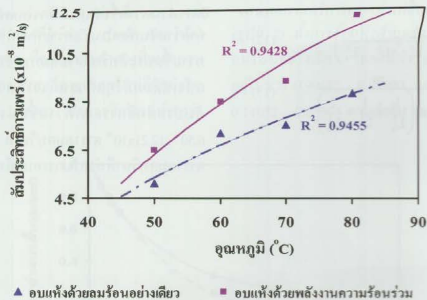
รูปที่ 5 สัมประสิทธิ์การแพร่ความชื้นประสิทธิภาพเมื่ออบแห้งเปลือกมังคุดด้วยพลังงานความร้อนร่วมและลมร้อนอย่างเดียว
