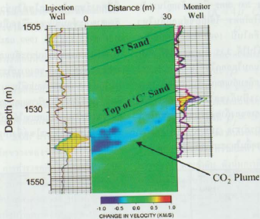
รูปที่ 9 แผนภาพโทโมกราฟี (กลาง) และข้อมูลความถี่ของคาร์บอนไดออกไซด์ในหลุมเจาะที่บ่อปั๊ม คาร์บอนไดออกไซด์ (ซ้าย) และบ่อเฝ้าติดตาม (ขวา) ขอบเขตของคาร์บอนไดออกไซด์ที่แผ่กระจายไป ระหว่างสองหลุมเจาะสอดคล้องกับความเร็วคลื่นต่ำ (สีฟ้า) (Daley et al., 2008)
