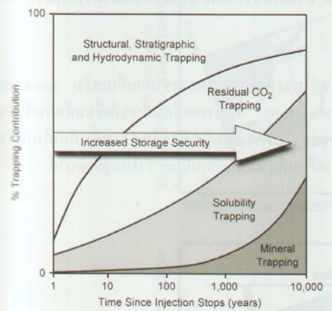
รูปที่ 3 ความปลอดภัยในการกักเก็บขึ้นอยู่กับกลไกการกักเก็บทางกายภาพและทางธรณีเคมี (IPCC, 2005)
