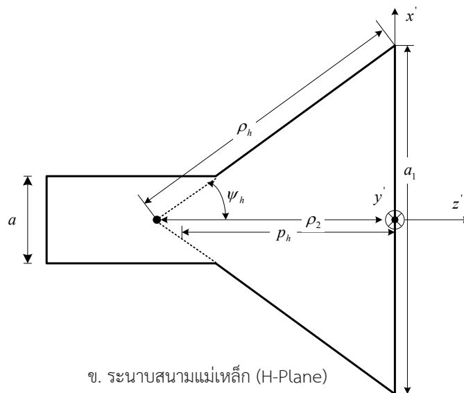
ภาพที่ 2 ค่าพารามิเตอร์สายอากาศปากแตรรูปพีระมิด ที่มา: Constantine, A. Balanis (2005)
