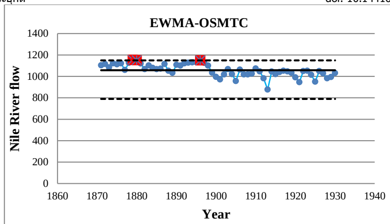
รูปที่ 7 ประสิทธิภาพการตรวจจับการเปลี่ยนแปลงค่าเฉลี่ยอัตราการไหลของแม่น้ำไนล์ตั้งแต่ปี 1871-1930 ระหว่างแผนภูมิควบคุม TCC , OSTC, EWMA-MTCC และแผนภูมิควบคุม EWMA-OSMTC (ต่อ)
