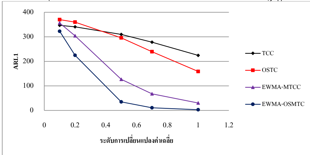
รูปที่ 6 ค่าความยาวรันเฉลี่ยของแผนภูมิควบคุม TCC, EWMA-MTCC, OSTC และแผนภูมิควบคุม EWMA-OSMTC ภายใต้ข้อมูลที่มีการแจกแจงลาปลาซ Laplace(1,1)
