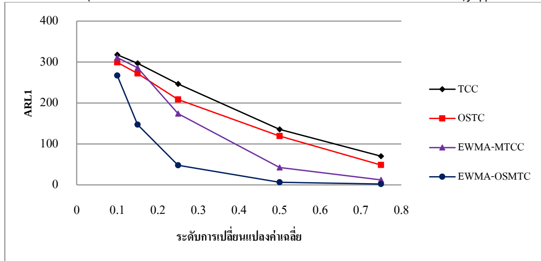
รูปที่ 4 ค่าความยาวรันเฉลี่ยของแผนภูมิควบคุม TCC, EWMA-MTCC, OSTC และแผนภูมิควบคุม EWMA-OSMTC ภายใต้ข้อมูลมีการแจกแจงปกติ Normal(0,1)
