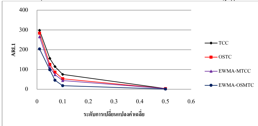
รูปที่ 5 ค่าความยาวรันเฉลี่ยของแผนภูมิควบคุม TCC , EWMA-MTCC, OSTC และแผนภูมิควบคุม EWMA-OSMTC ภายใต้ข้อมูลที่มีการแจกแจงไวส์บูล Weibull(3.5,1)
