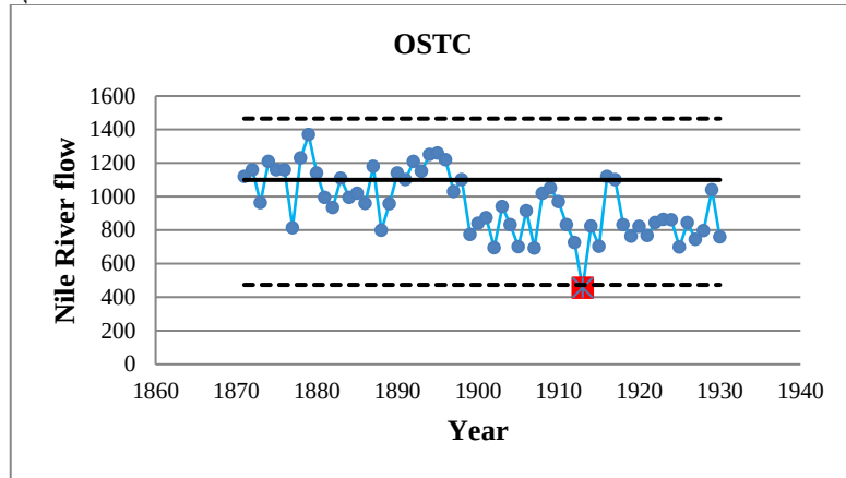
รูปที่ 7 ประสิทธิภาพการตรวจจับการเปลี่ยนแปลงค่าเฉลี่ยอัตราการไหลของแม่น้ำไนล์ตั้งแต่ปี 1871-1930 ระหว่าง แผนภูมิควบคุม TCC, OSTC, EWMA-MTCC และแผนภูมิควบคุม EWMA-OSMTC
